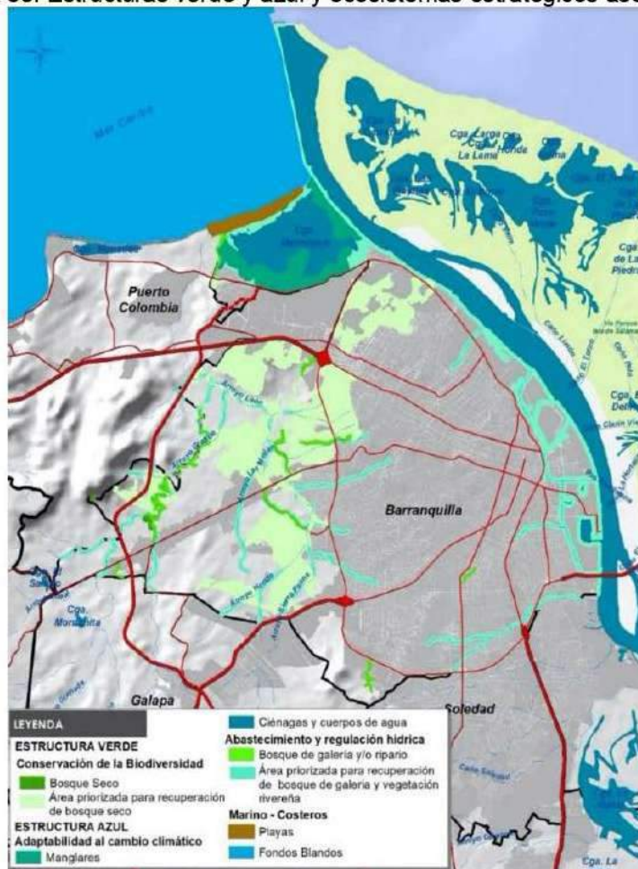
Figura 85. Estructuras verde y azul y ecosistemas estratégicos asociados.
