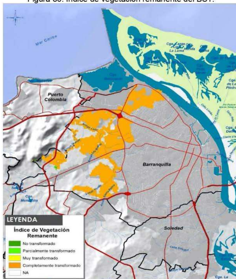
Figura 86. Índice de vegetación remanente del BST.
