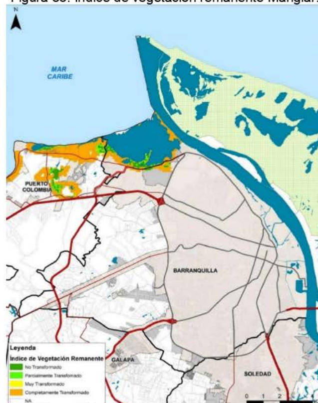
Figura 88. Índice de vegetación remanente Manglar.
