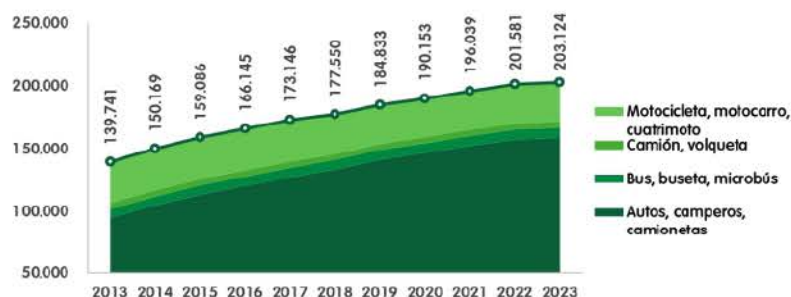
Figura 69. Crecimiento histórico del parque automotor en el Distrito de Barraquilla.
