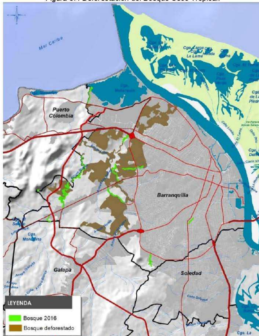
Figura 87. Deforestación del Bosque Seco Tropical.
